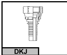
DKJ HEMBRA JIC cono 74° JIC FEMALE 74° cone
