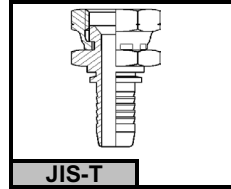
JIS-T HEMBRA JIS (T) cono 60° JIS FEMALE (T) 60° cone
