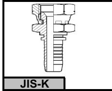
JIS-K HEMBRA JIS (K) cono 60° JIS FEMALE (K) 60° cone
