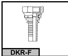
DKR-F HEMBRA GAS serie plana BSP FEMALE flat face
