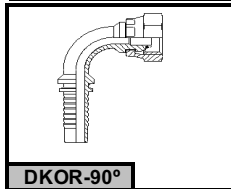
DKOR-90° CODO GAS A 90° cono 60° con junta 90° BSP SW.ELBOW 60° cone o-ring
