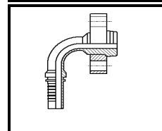
BRIDA POCLAIN 90° GIRATORIA POCLAIN FLANGE 90° SWIVEL
