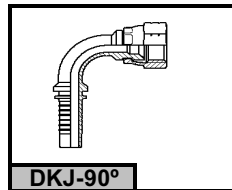
DKJ-90° CODO JIC A 90° cono 74° 90° JIC SW.ELBOW 74° cone
