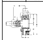
113102 TE ORIENTABLE EN L JIC GAS CILINDRICO JUNTA
