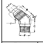
105048 CODO 45° JIC NPTF
