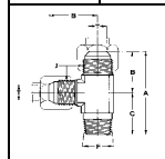
113047 TE ORIENTABLE EN L JIC NPTF
