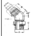
105037 CODO 45° ORIENTABLE JIC METRICO CIL. JUNTA
