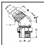
105026 CODO 45° ORIENTABLE JIC GAS CILINDRICO JUNTA
