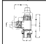
113036 TE ORIENTABLE EN L JIC METRICO CIL. CON JUNTA
