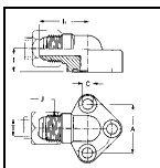
407124 MANGUITO 90° MACHO JIC REFORZADO
