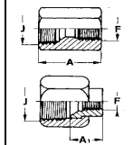
102298 RACOR MANOMETRO HEMBRA JIC HEMBRA GAS CILINDRICO
